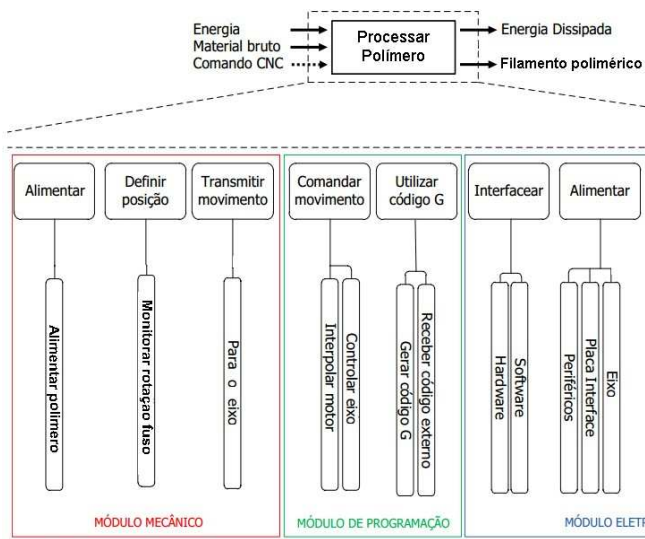
Figura 1: Síntese funcional para o módulo extrusor.
