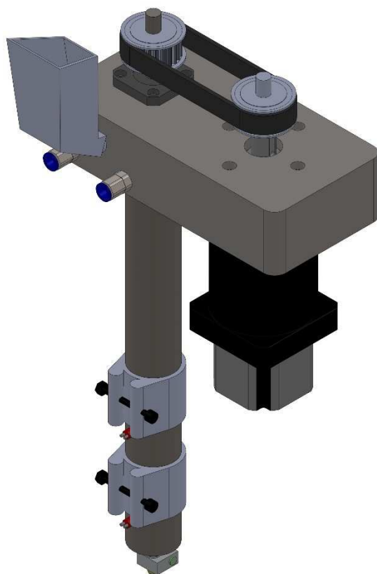
Figura 3: Montagem em CAD do módulo extrusor.
