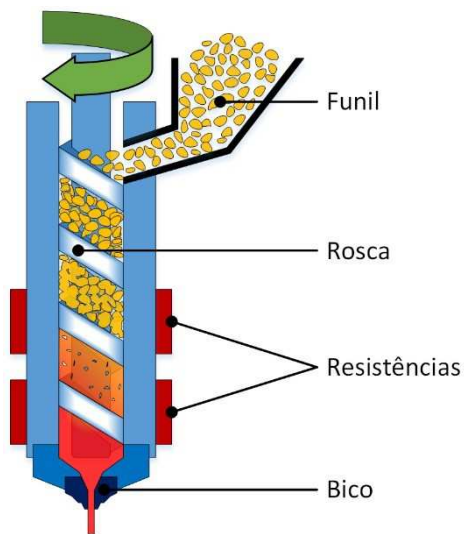
Figura 2: Esquema do módulo extrusor com os principais componentes.
